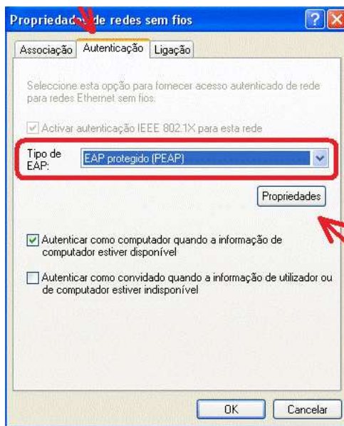
Figura 6 - Tipo de autenticação.
