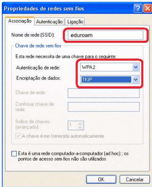
Figura 5 - Definições de encriptação.
